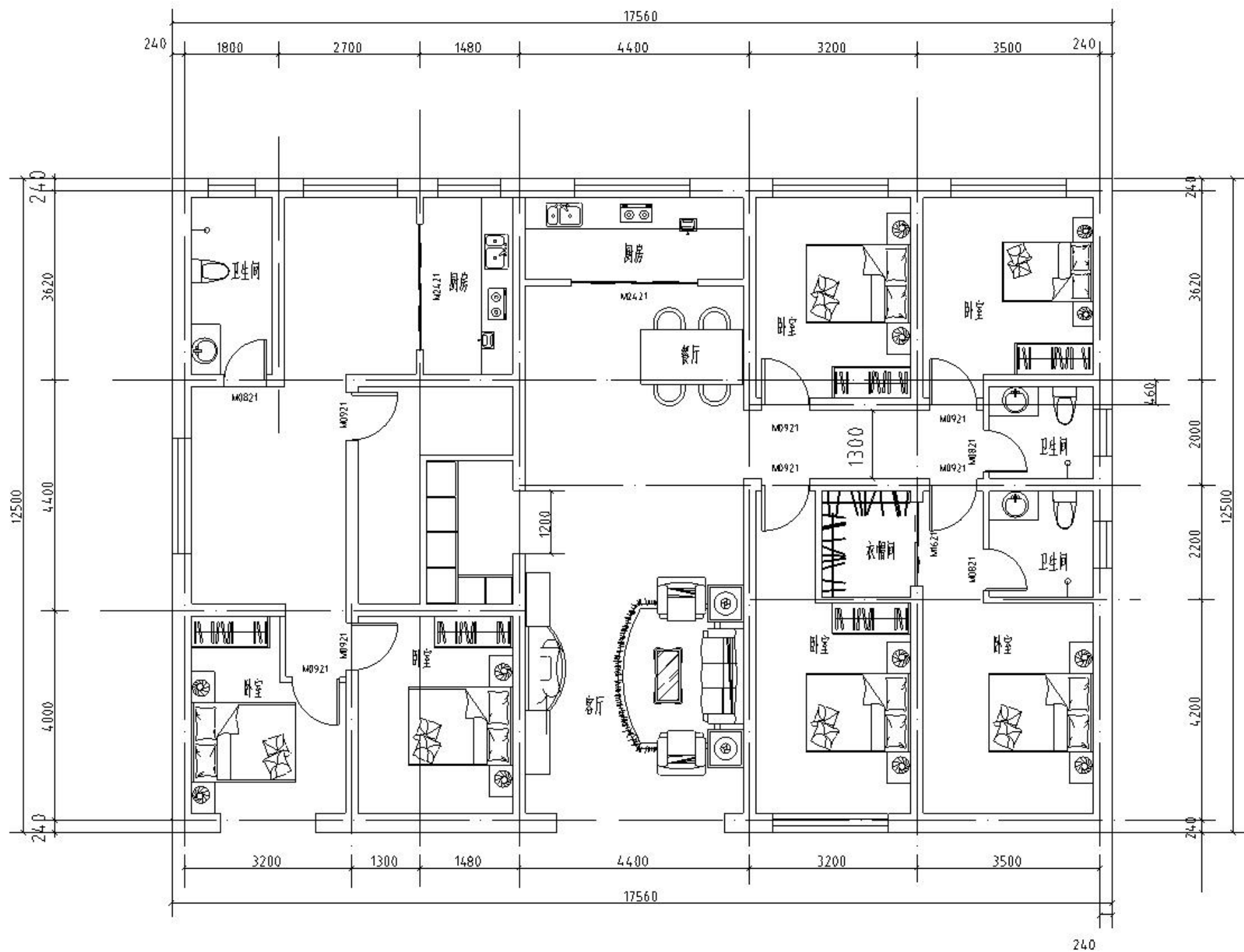
一层平面图 1:100
